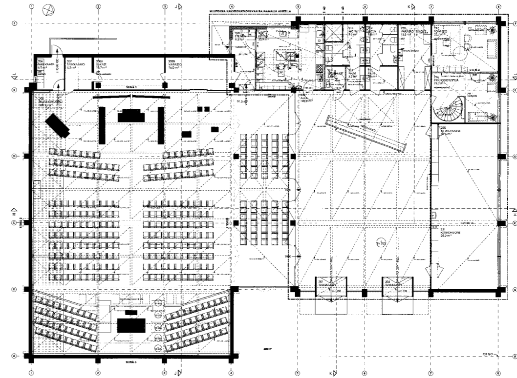
Liipolan seurakuntakeskuksen pääkerroksen pohjapiirros. Vasemmalla näkyy kirkkosali.
